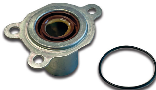
Image 1 : Douille de guidage Réf. 414 0024 10 avec joint d'étanchéité séparé
