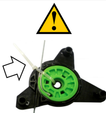
POWER WINDOW LEFT ALZACRISTALLI ELETTRICO SX
